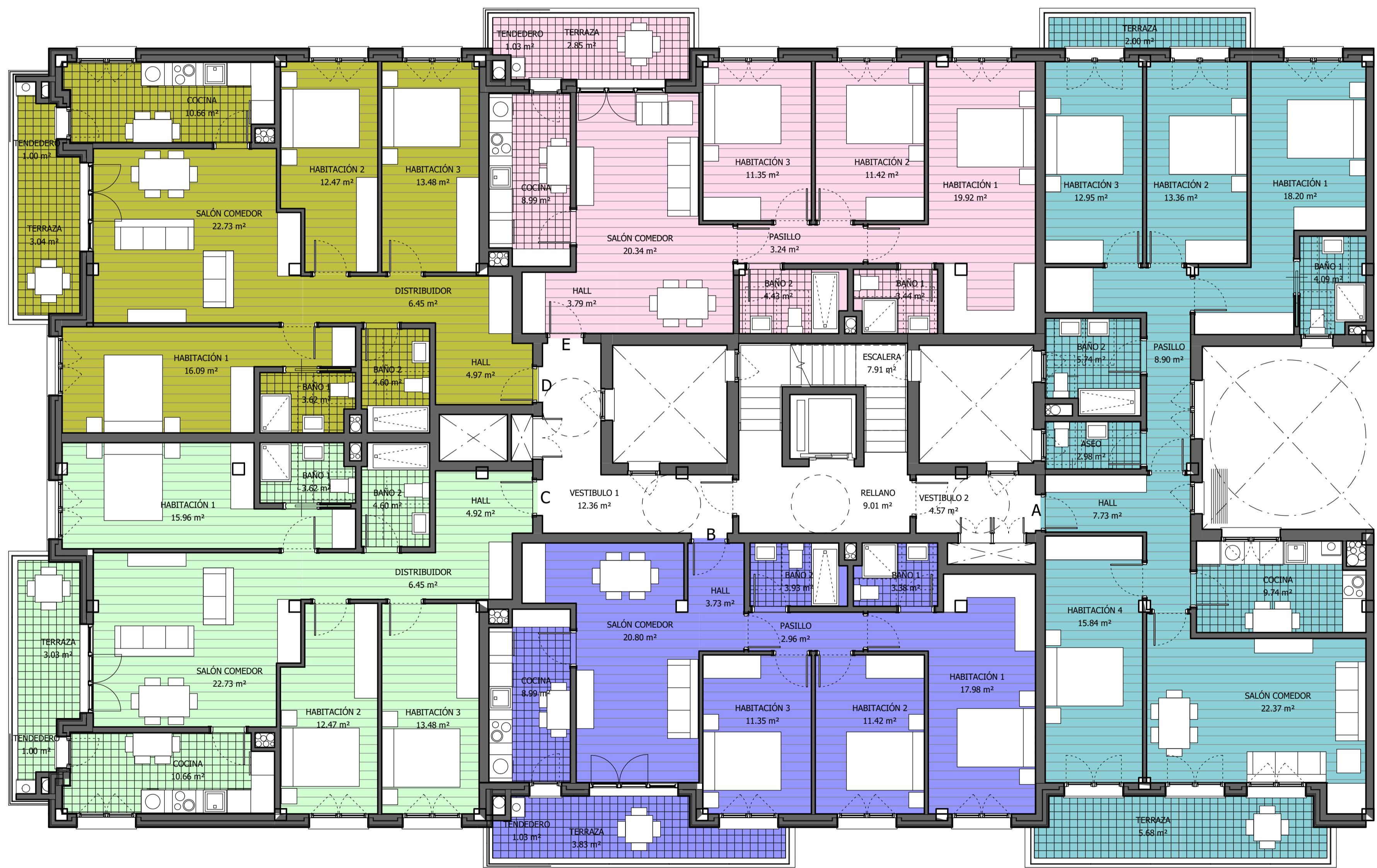
P.01 PLANTA 1º 1:75
