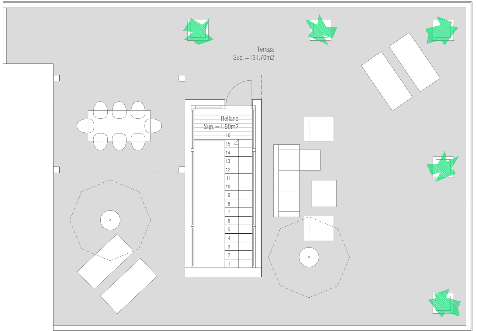
PLANTA DE CUBIERTAS E 1:75
